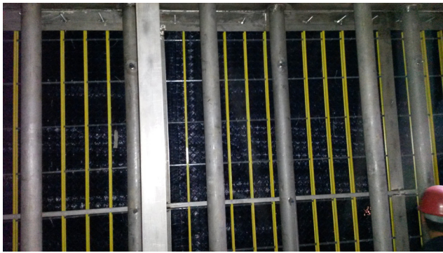
Рисунок 1. Сеточные прокладки BlueFil® из структурированного полипропилена, обрабатывающие выбросы гранулятора и охладителя до <math>< 30 \text{ mg/Nm}^3</math>
