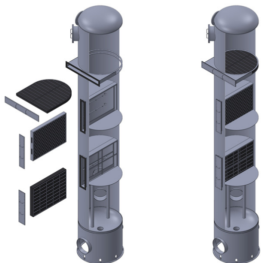
Рисунок 4. Сетка BlueFil MX095 из полипропилена
